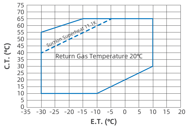
YM34-115 R452A
