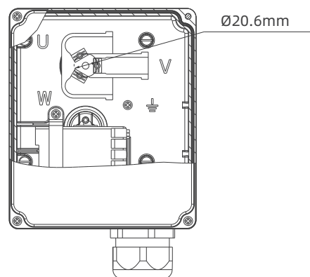
T-Box Layout
